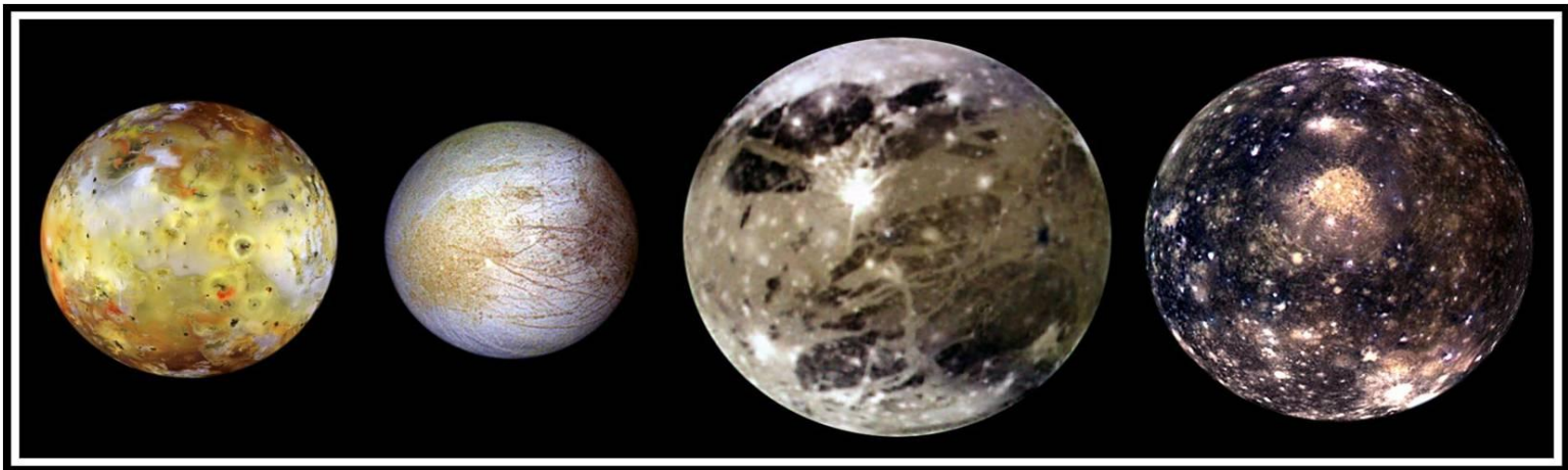
Io
