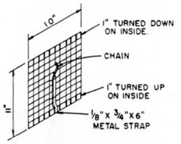
DOOR DETAILS
